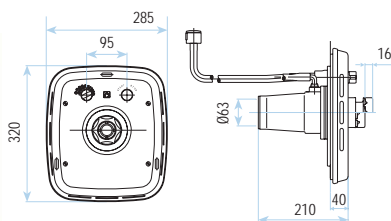
Plástico branco para caixa de alojamento em inox (Cód. 11501) White ABS for S.S. wall housing (Cod. 11501)
