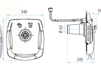
Com pega incluída em plástico branco para caixa de alojamento de plástico (Cód. 11013) Built-in hand grip in white plastic for plastic wall housing (Cod. 11013)
