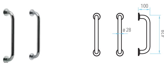
Dupla em inox AISI-316 polido (Cód. 05557) S.S. AISI-316 polished for twin faceplate (Cod. 05557)
