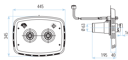
Rectangular dupla em plástico branco (Cód. 11508) Twin faceplate in white plastic (Cod. 11508)
